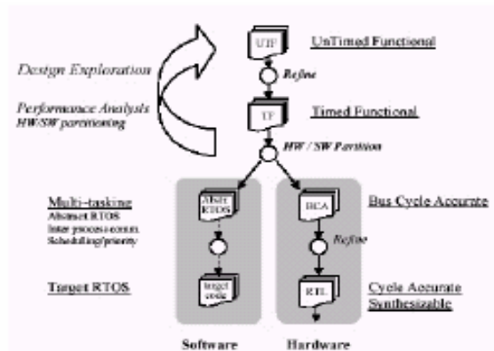
Figure 1 : Niveaux d'abstraction : SystemC
